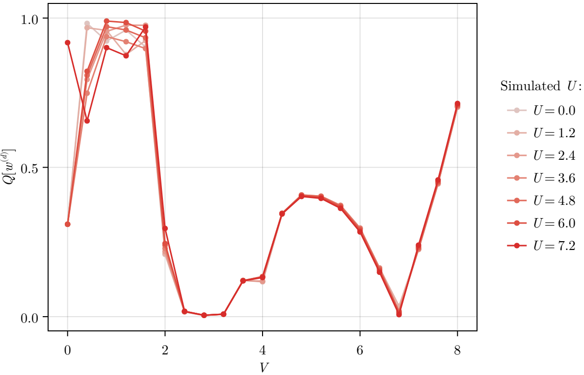
Q[w^{(d)}] \text{ } (t=1.0, L=256, \delta=0.0, \beta=100.0)
